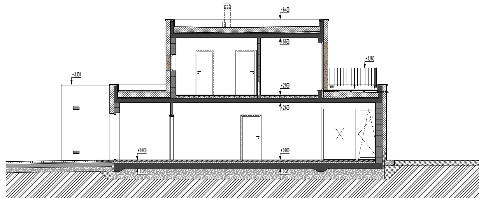
POZDĽŽNY REZ CC/ LONGITUDAL - SECTION CC
