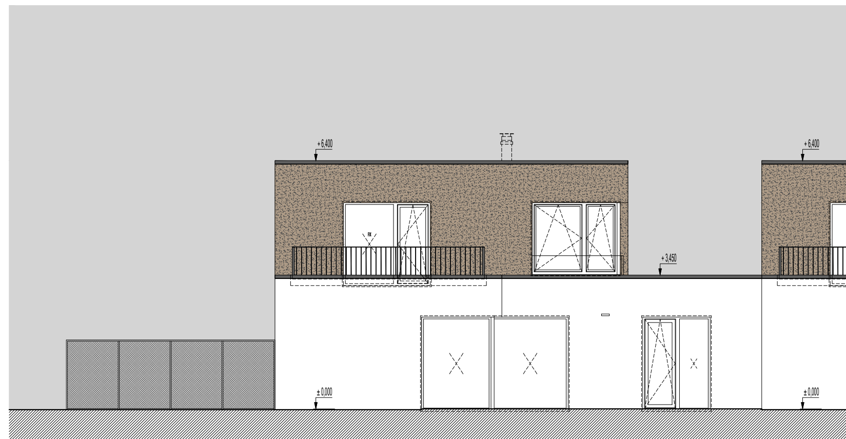
POHLAD 02 - OD ZÁHRADY/ GARDEN ELEVATION
